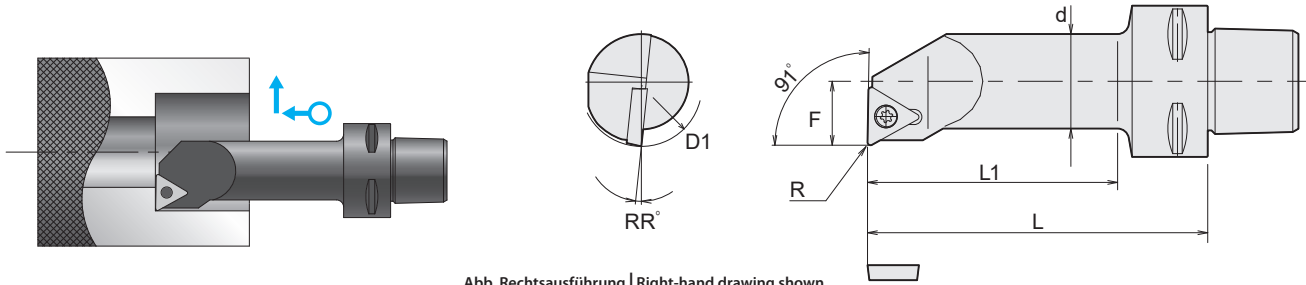
Abb. Rechtsausführung | Right-hand drawing shown
