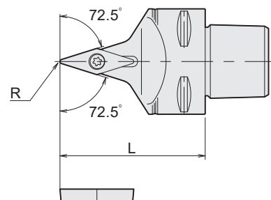
Abb. Rechts- und Linksschneidend For both Right and Left-hand.
