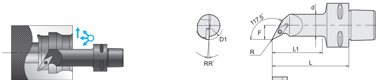
Abb. Rechtsausführung | Right-hand drawing shown
