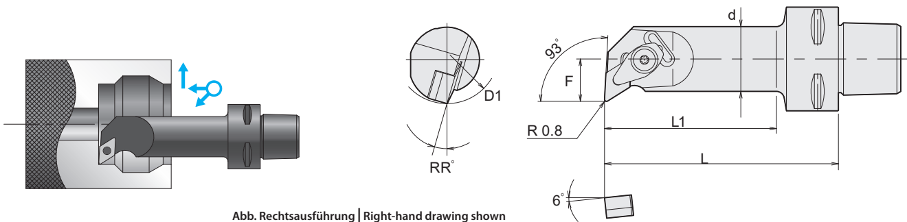
Abb. Rechtsausführung | Right-hand drawing shown
