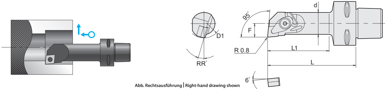
Abb. Rechtsausführung | Right-hand drawing shown
