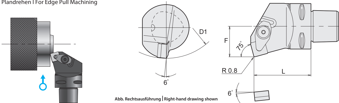
Abb. Rechtsausführung | Right-hand drawing shown
