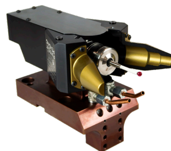
MT-TPS SONDA DE MEDICIÓN
