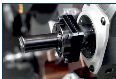
MICRO REGULACIÓN EN "Y" (OPCIONAL)
