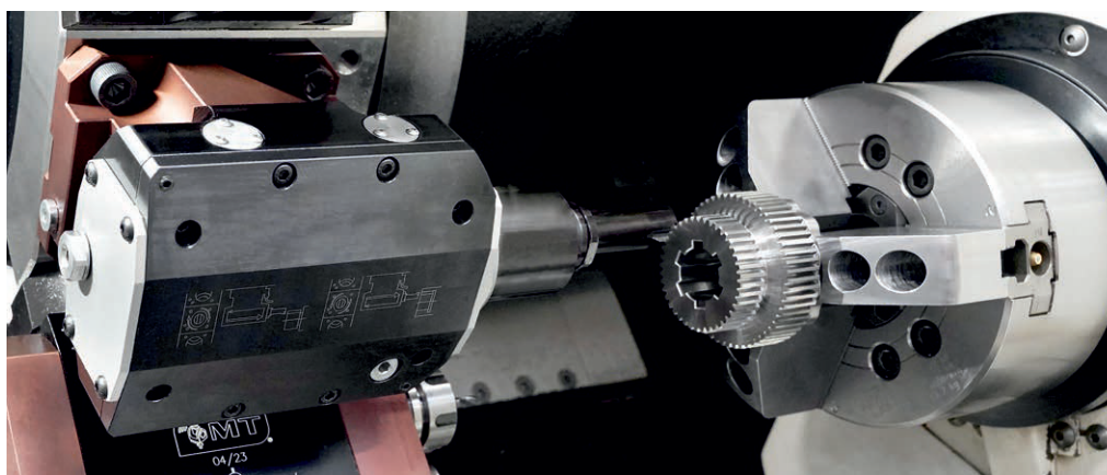
ENGRANAJE EXTERIOR
