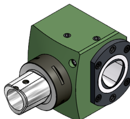
ADAPTADOR CAPTO A CAPTO
