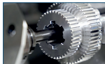
CHAVETERO
